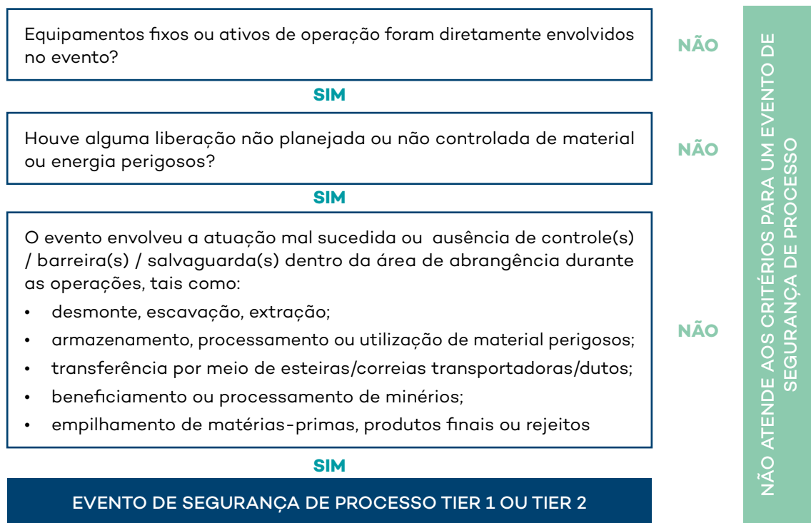
Figura 2: Fluxograma de Identificação de Evento de Segurança do Processo
